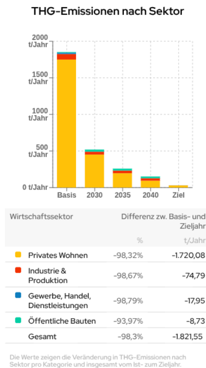
Abbildung 25: Zielszenario – Entwicklung Treibhausgasemissionen
