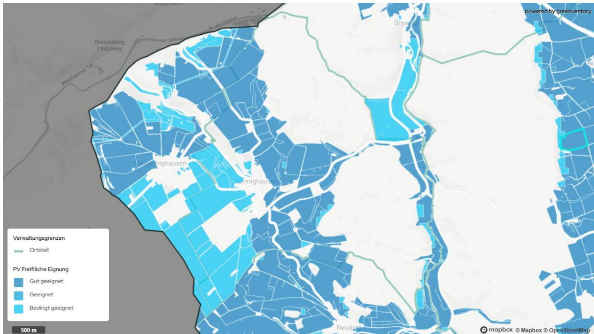
Abbildung 13: Potenzial für Freiflächen-Photovoltaik
