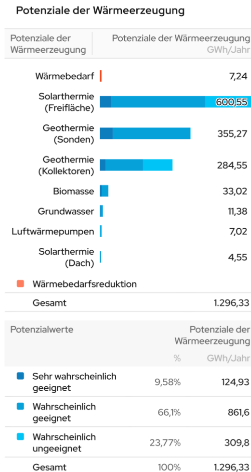
Abbildung 15: Potenziale zur Wärmeerzeugung und Wärmereduktion
