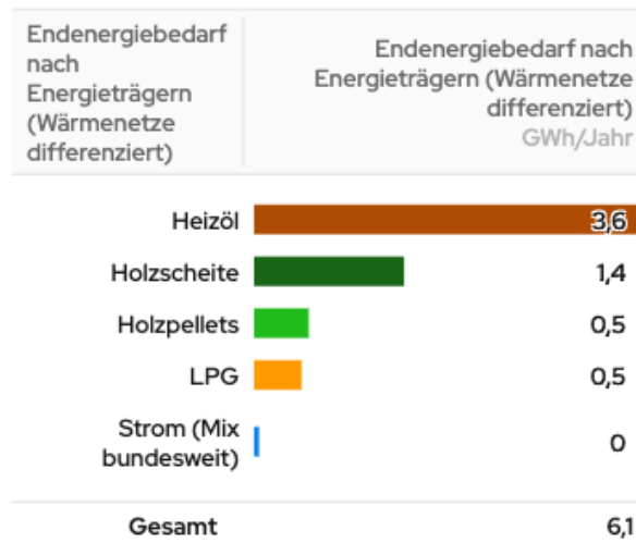
Abbildung 9: Endenergiebedarf nach Energieträgern
