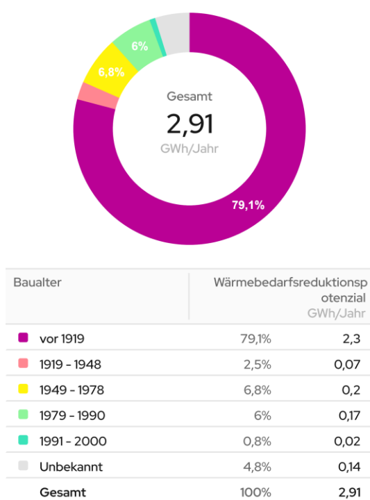
Abbildung 19: Sanierungspotenzial nach Gebäudealter
