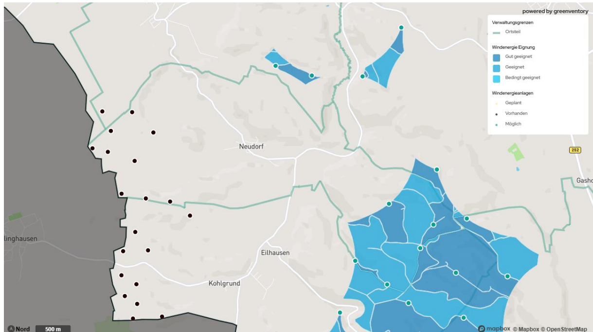
Abbildung 14: Potenzial für Windenergieanlagen
