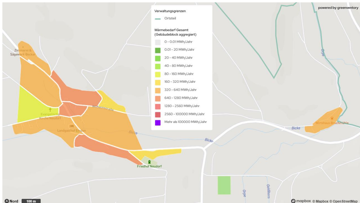
Abbildung 4: Wärmebedarf absolut
