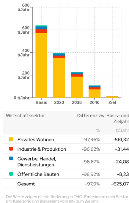
Abbildung 25: Zielszenario - Entwicklung Treibhausgasemissionen
