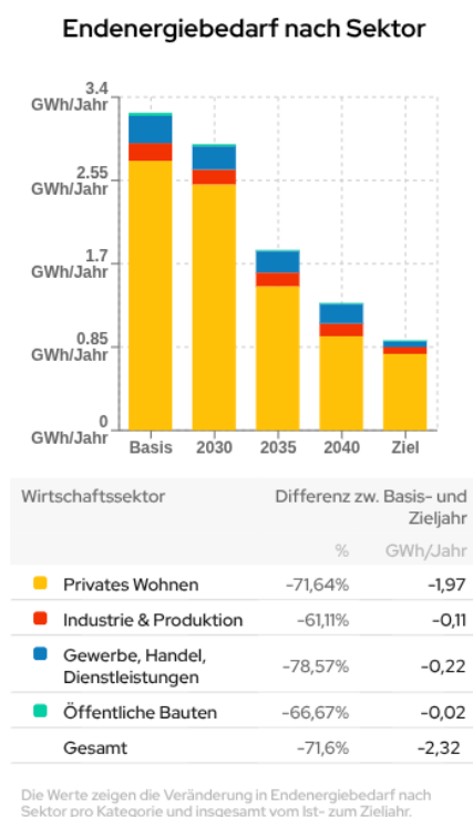
Abbildung 22: Zielszenario – Entwicklung Endenergiebedarf nach Sektoren
