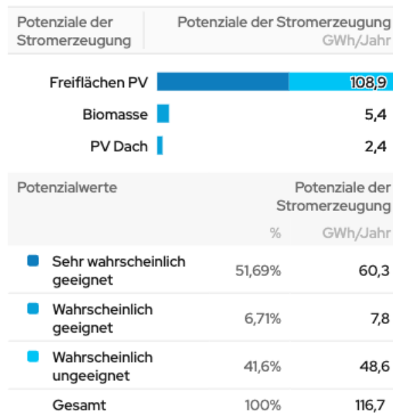
Abbildung 12: Potenziale zur Stromerzeugung
