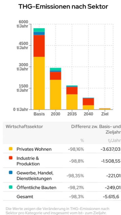
Abbildung 26: Zielszenario – Entwicklung Treibhausgasemissionen
