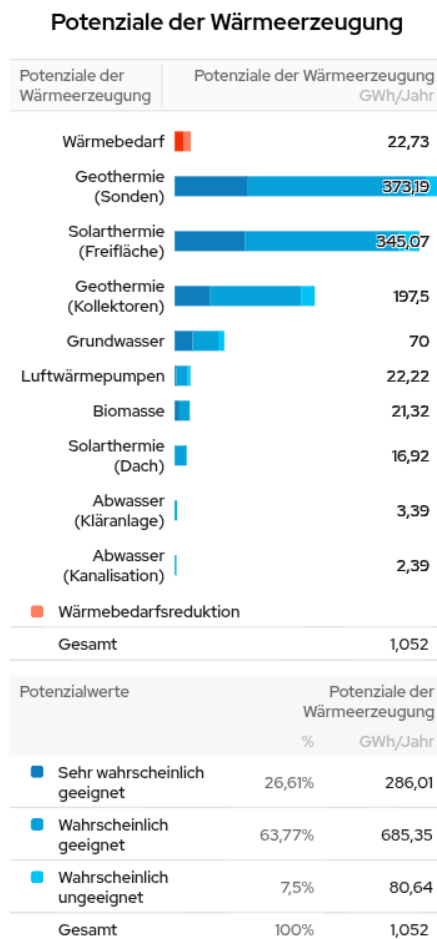
Abbildung 16: Potenziale zur Wärmeerzeugung und Wärmereduktion
