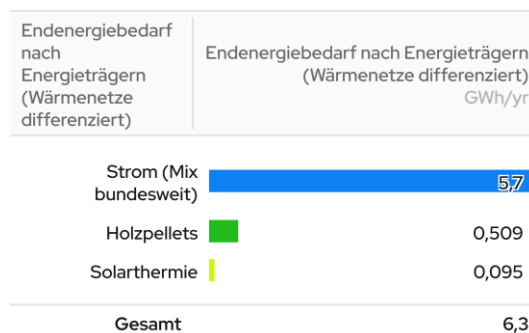
Abbildung 24: Zielszenario – Endenergiebedarf nach Energieträgern
