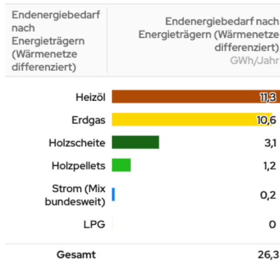
Abbildung 9: Endenergiebedarf nach Energieträgern
