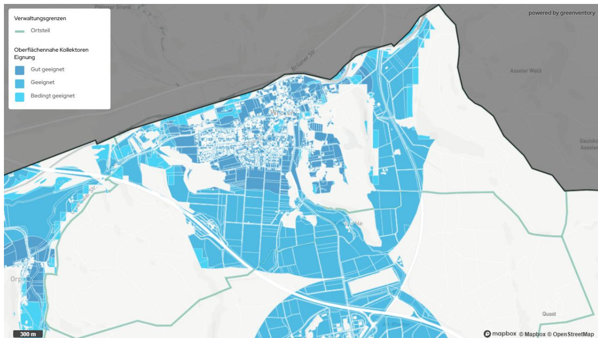
Abbildung 19: Geothermie-Eignung Kollektoren
