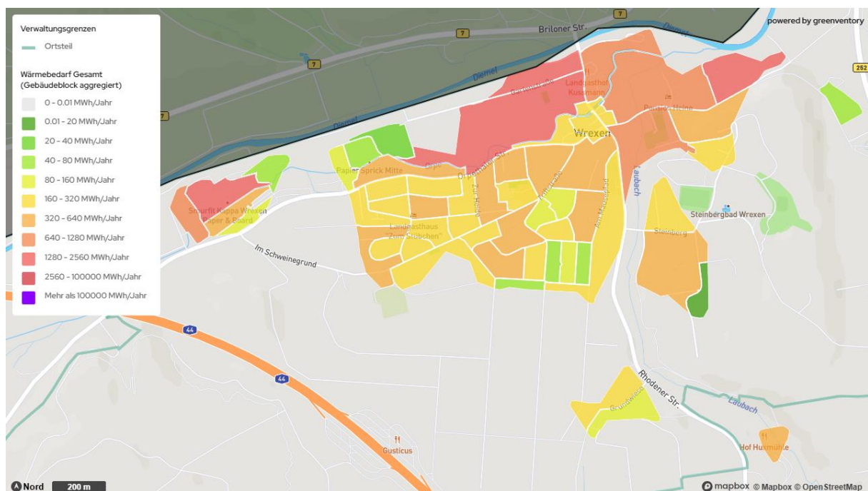
Abbildung 4: Wärmebedarf absolut
